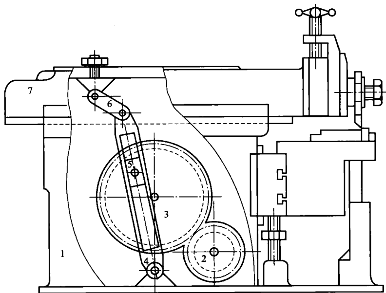
图 1-1 牛头刨床
