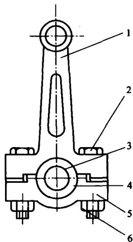
图 1-2 连杆
