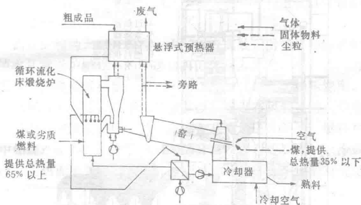
图 1.2 制水泥用的循环流化床预煅烧炉
