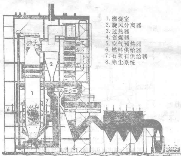
图1.3 循环流化床锅炉示意图
