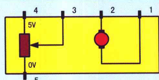
风板电动机
