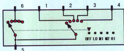
鼓风机调速开关
