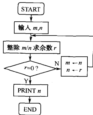
图 1.7 算法的框图描述
