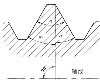
图 1-15 螺纹牙侧角
