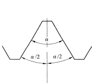
图 1-14 螺纹牙型角和牙型半角
