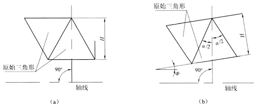
图 1-8 螺纹原始三角形
