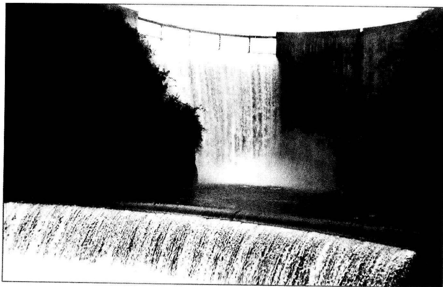
黔南州“九五”期间的重要水利工程猛坑水库大坝溢洪的壮观场景
