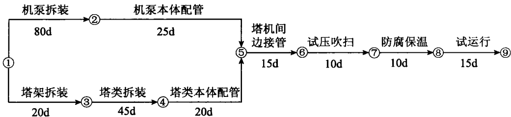
图 1-2 重编的网络计划
