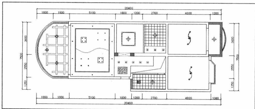
一层天棚图.....282
