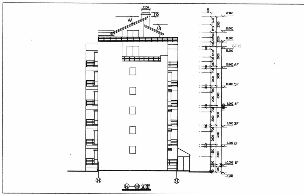
小区高层住宅立面图 3.....348
