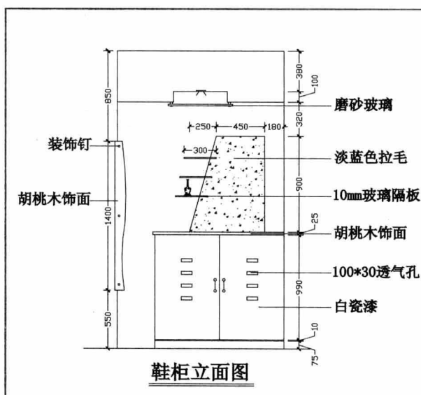
鞋柜立面图.....195
