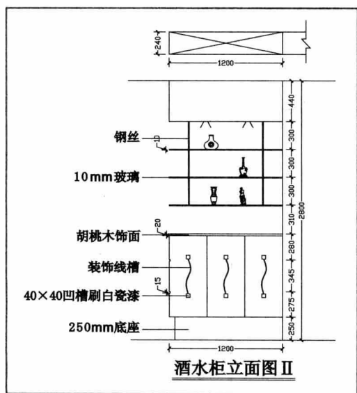
酒柜立面图.....195
