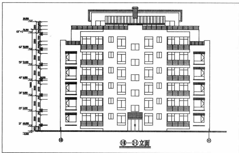
小区高层住宅立面图 1.....348
