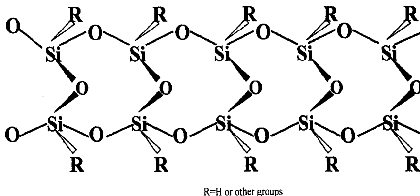
反应性梯形高分子结构示意图
