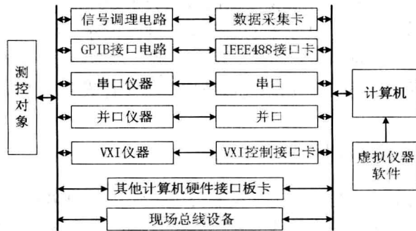
图 1-2 虚拟仪器结构框图
