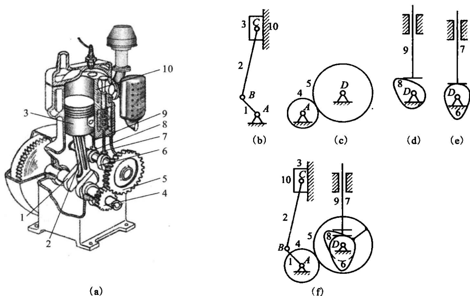
图 1-1 立式单缸内燃机
