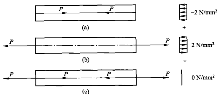
图 1-1 轴心受拉构件在预加应力前后截面应力变化示意图
