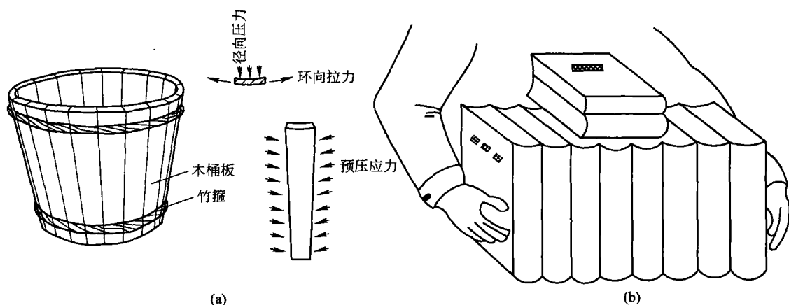
图 1-3 采用预压应力的生活实例
