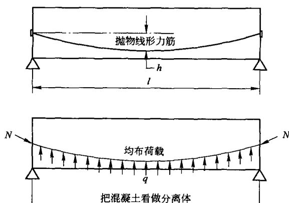
图 1-6 抛物线配筋的简支梁
