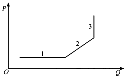
图 1—2 总供给曲线
