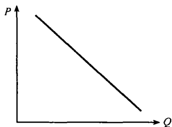
图 1—3 总需求曲线
