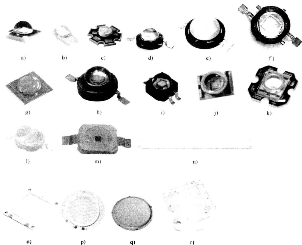
图 1-4 High Power（大功率）系列 LED 外形
