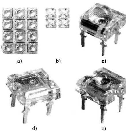
图 1-3 食人鱼系列 LED 外形
