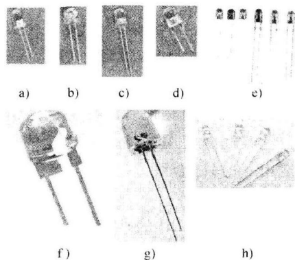
图 1-1 Lamp 系列 LED 外形
