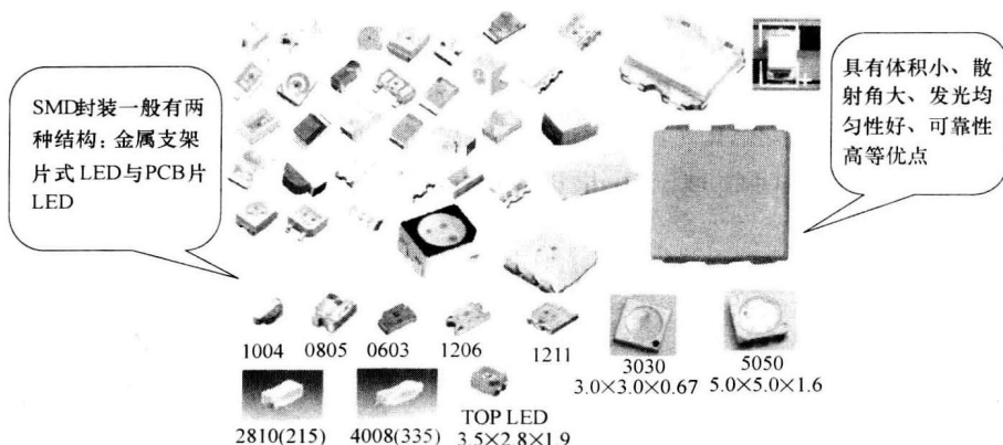
图 1-2 TOP 系列 LED 外形
