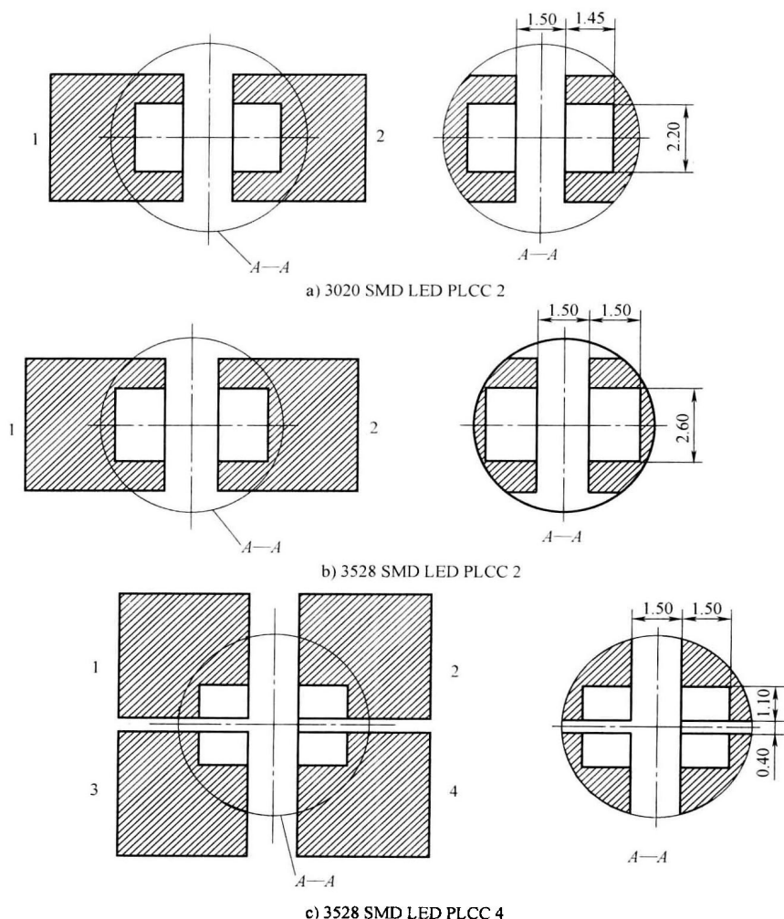
图 1-7 TOP LED 元件焊盘散热设计
