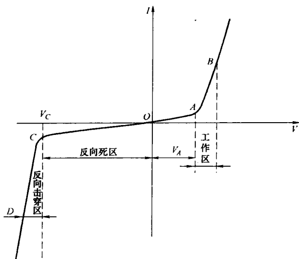
图 1-5 LED 的伏安特性曲线
