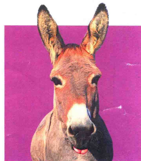
毛驴 donkey
