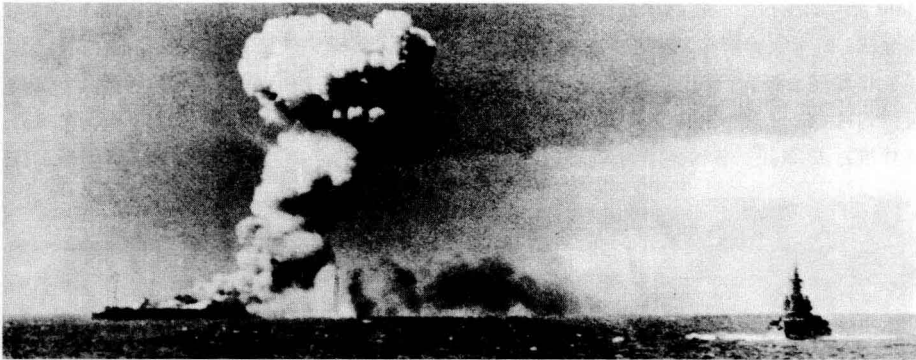
“普林斯顿”号在“神风”突击队自杀性攻击下走火，其右侧为美军重型巡洋舰“瑞诺”号。
