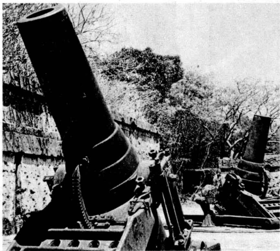
12英寸口径的迫击炮阵地。
