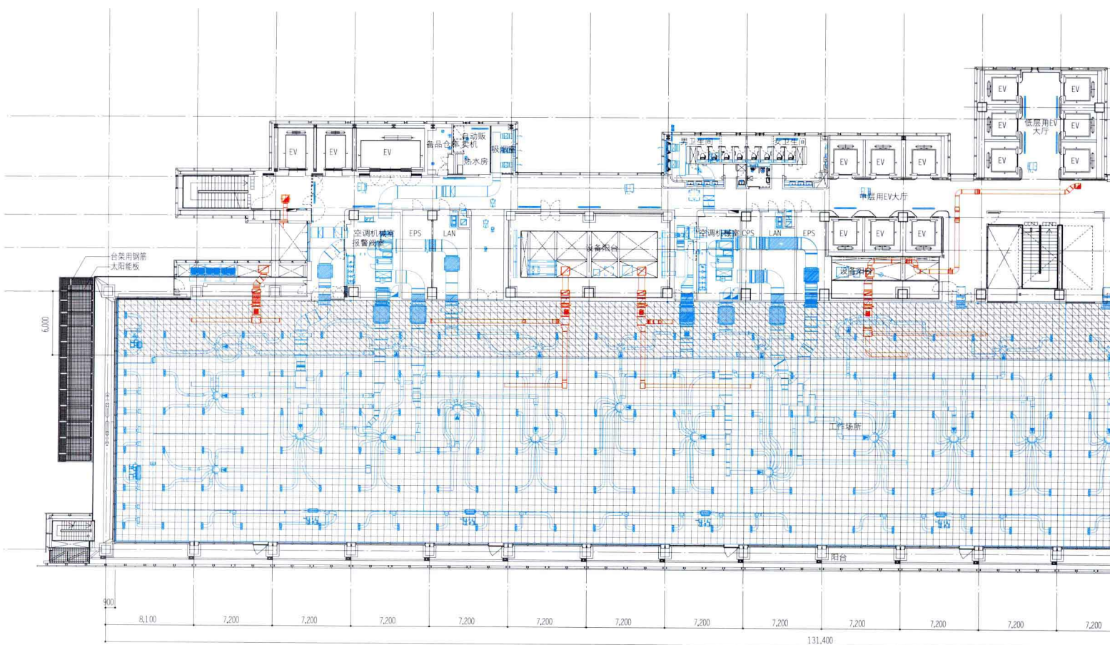
标准层平面图 比例1/500 (图面颜色显示了吊顶背面的设备。蓝色为空调设备, 红色为排烟设备。)
