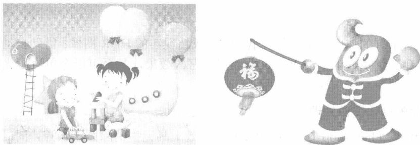
图 1-5 卡漫设计
