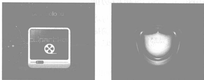
图 1-4 界面设计
