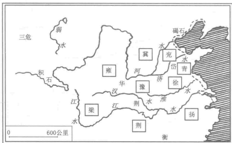
图 0-2 上古时期“九州”位置示意图
