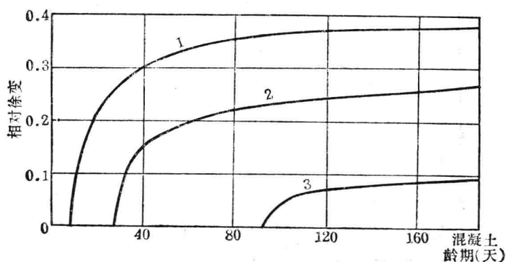
图 1-9 加荷时混凝土龄期与相对徐变的关系
