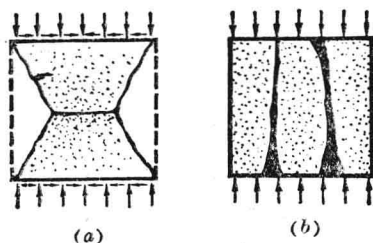
图 1-1 立方体试件破坏情况 (a) 支承面上有摩擦力存在；(b) 支承面上 无摩擦力存在(涂有油脂)
