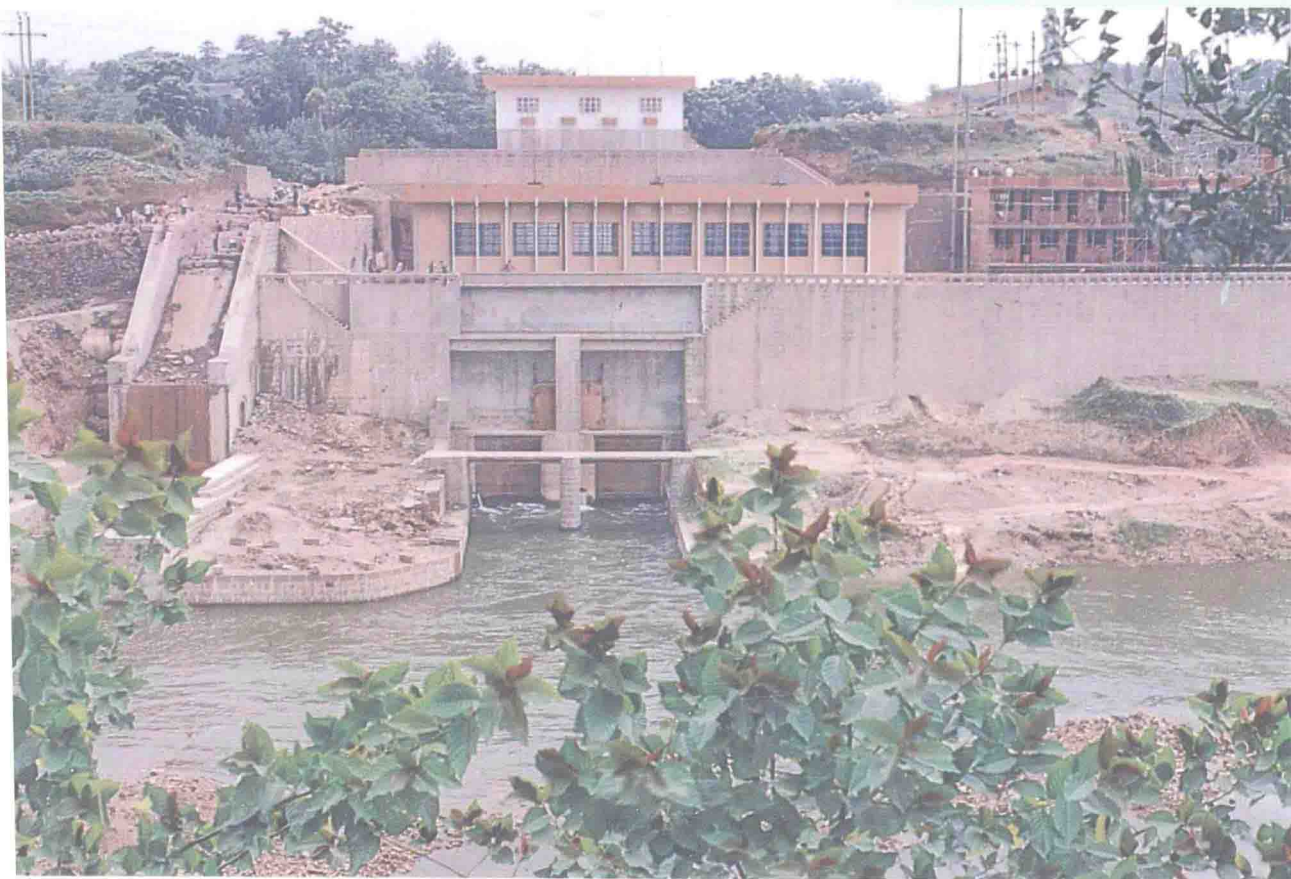
图为即将建设竣工的潼南县高肯调峰水电站外景。
