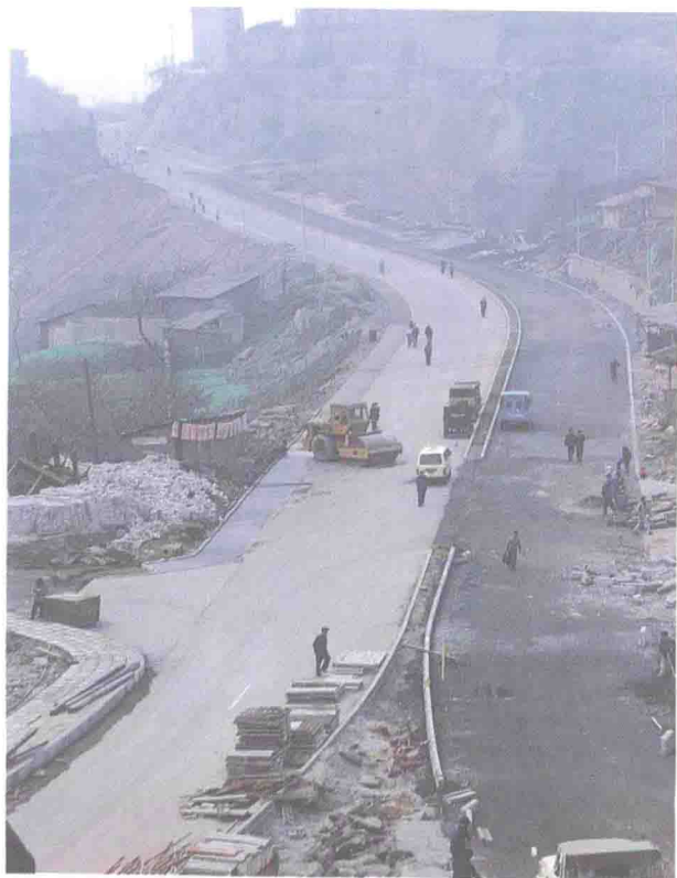
图为建设中的菜袁公路中段。
