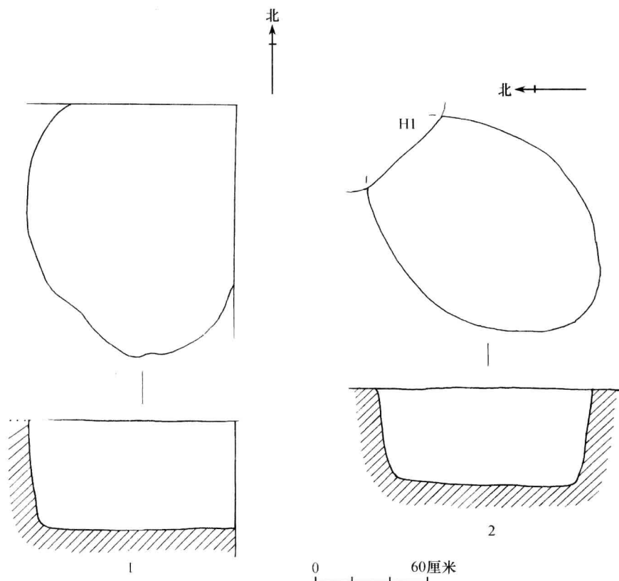
图四 H1、H8 平、剖面图
