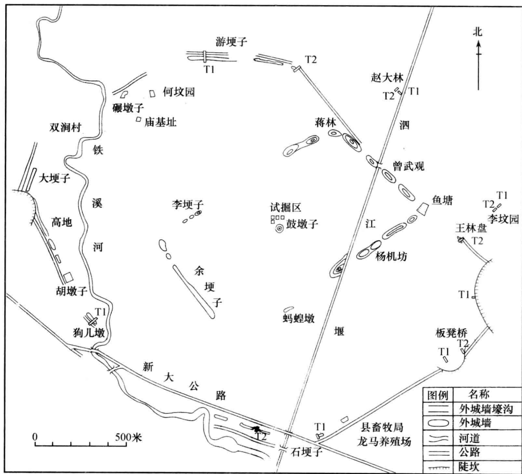
图二 宝墩遗址平面图
