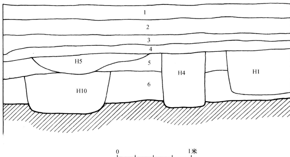
图三 T2431北壁剖面图
