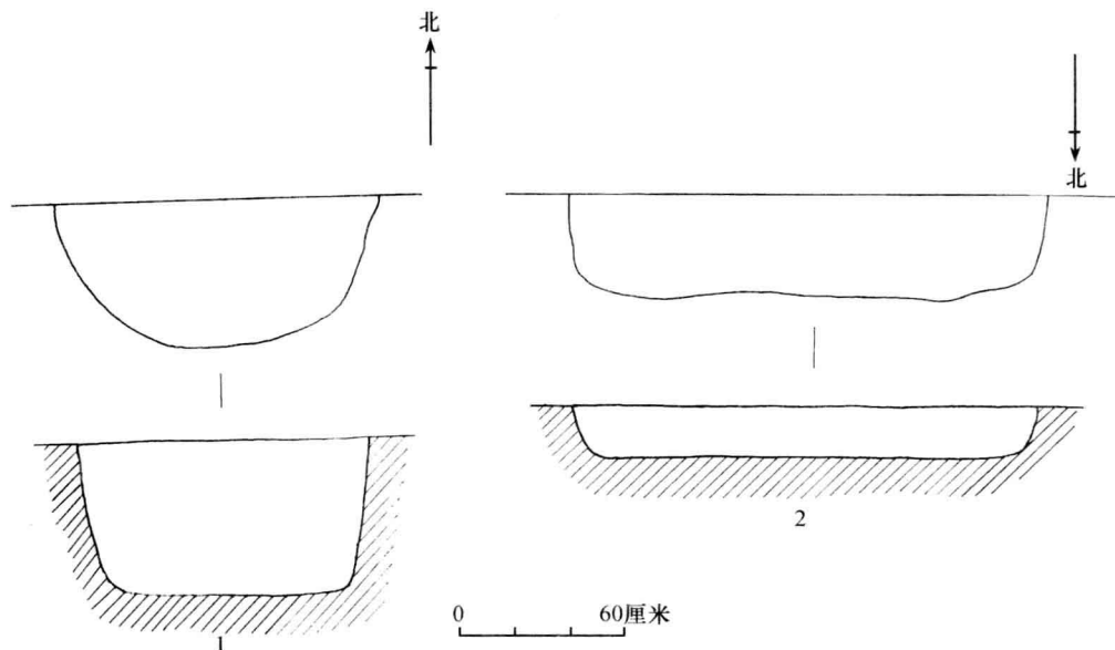
图五 H3、H10 平、剖面图
