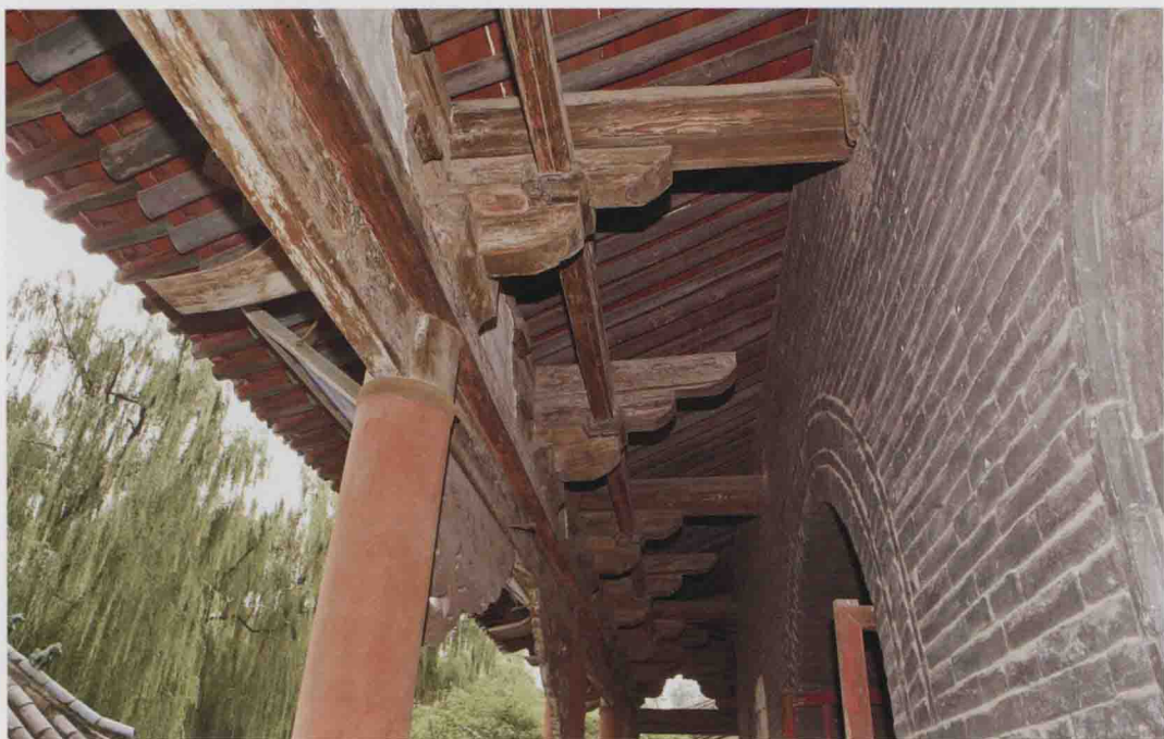
晋祠水母楼一层外廊构造
