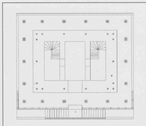
晋祠水母楼一层平面示意图
