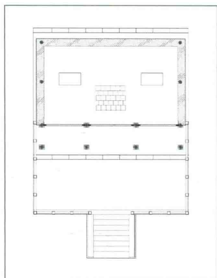
晋祠贞观宝翰亭平面示意图
