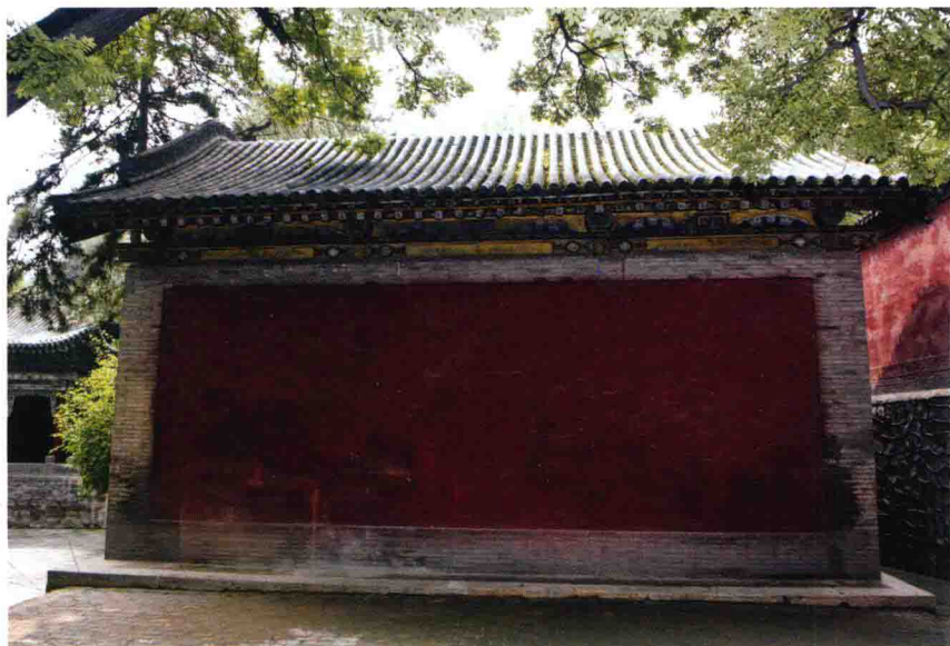
晋祠贞观宝翰亭背立面
