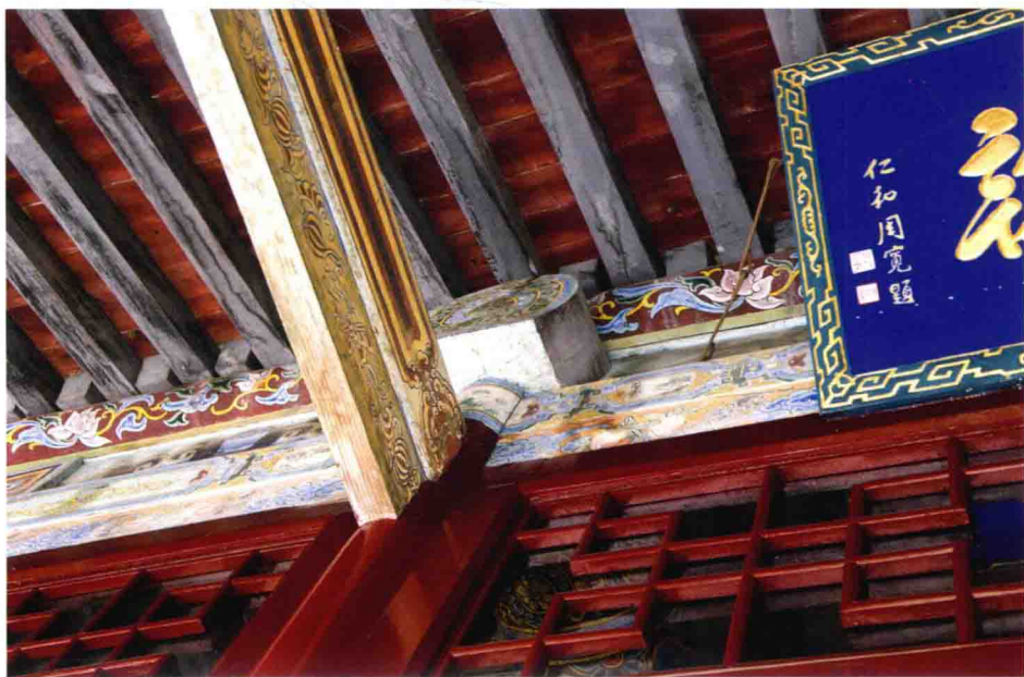
晋祠贞观宝翰亭柱、梁节点
