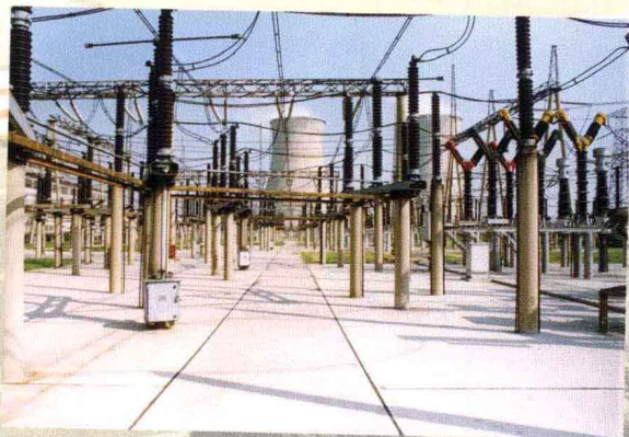
220kV变电所
