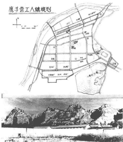
图 1-3 鹰手营工人镇规划
