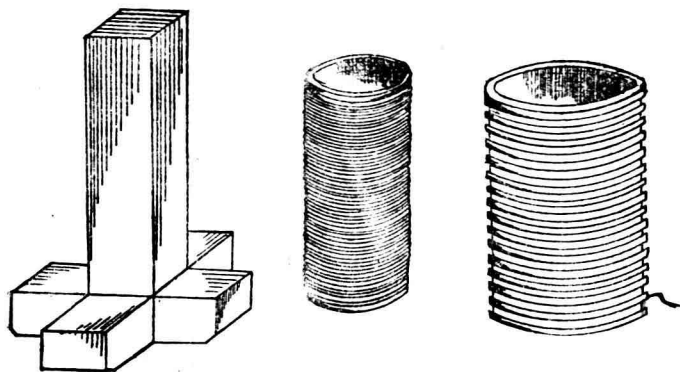
圖 7 大容量四部分佈芯式變壓器的鐵芯與線捲
