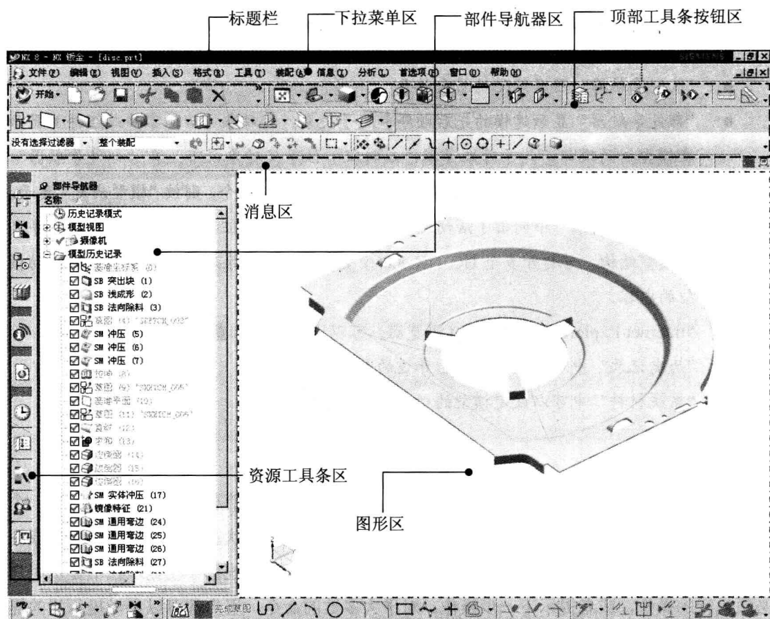
图 2.1.1 UG NX 8.0 钣金设计模块工作界面
