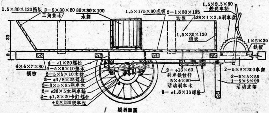
縱剖面圖
