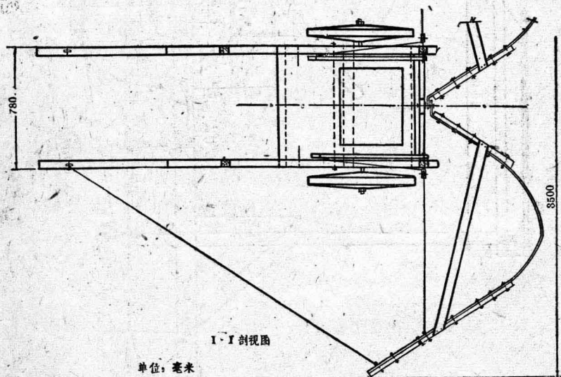
畜力双边杠杆式回砂車①
