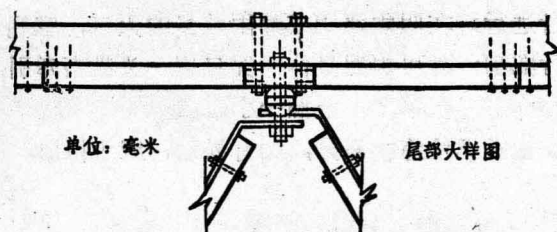
畜力双边杠杆式回砂車③
