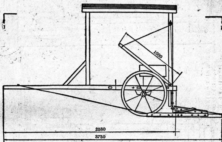
侧面图
