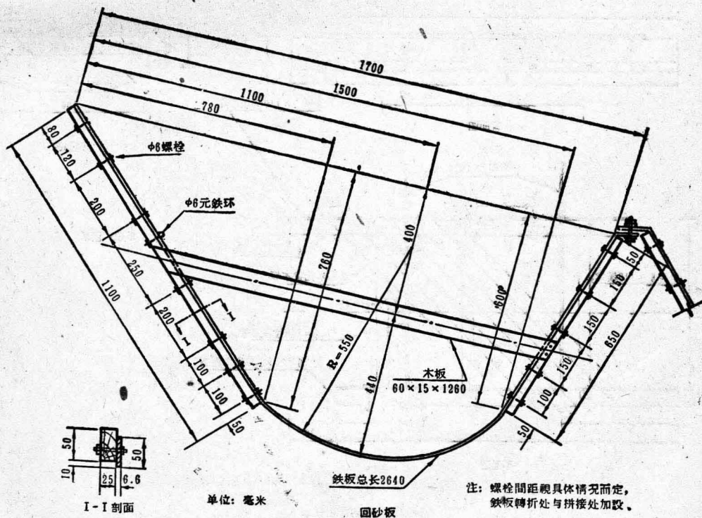
畜力双边杠杆式回砂車④
