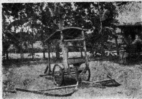
畜力双边杠杆式回砂車回砂板升起情况
