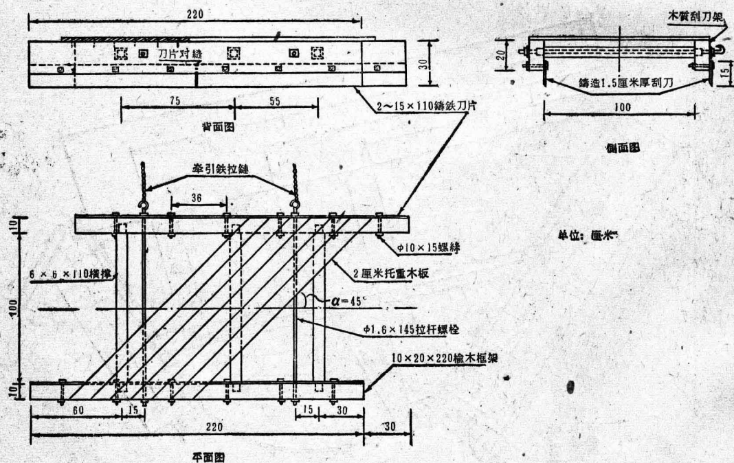
畜力路拖子
