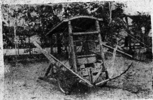
畜力双边杠杆式回砂車全貌
