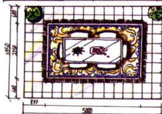
餐厅平面图 1:50
