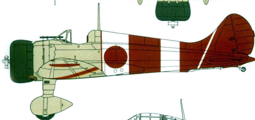
96式4号舰战全身涂 装侧视图，1939年11 月，航母赤城战斗 机队。机翼上的红黄 相间条纹表明这是 飞行队长座机。机身 为浅灰色。
