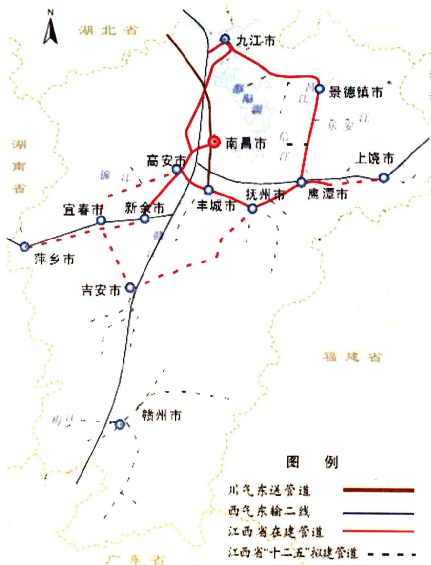
图9 天然气管网规划图
