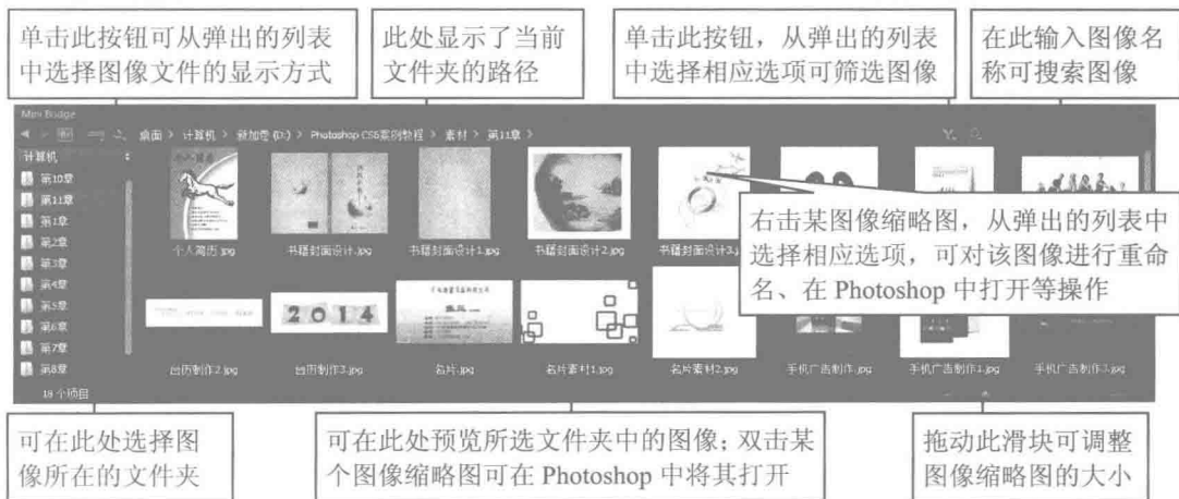
图 1-17 Mini Bridge
