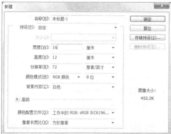
图 1-21 “新建”对话框
