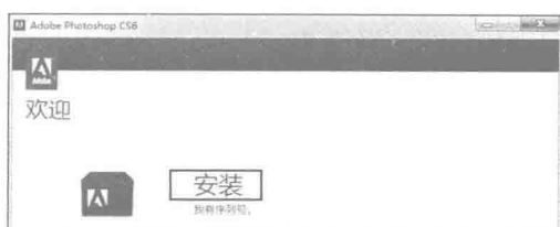
图 1-2 “欢迎”对话框
