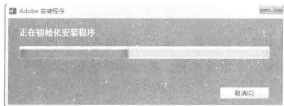
图 1-1 初始化安装
