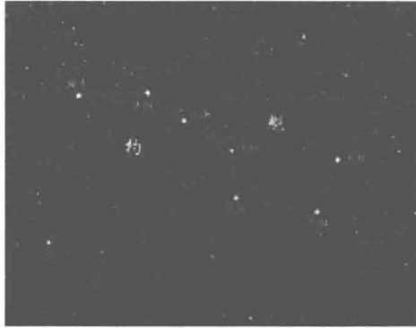
图 1-1 北斗星座图
