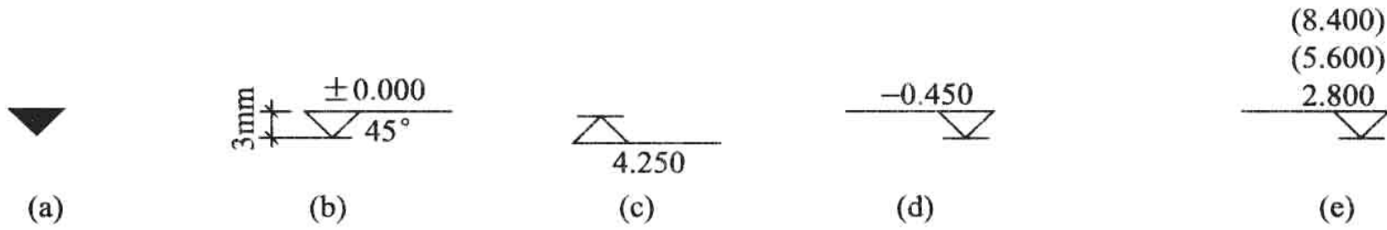
图 1-9 标高数字的注写
