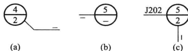
图 1-6 用于索引剖面详图的索引符号
