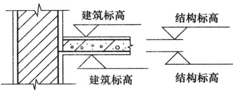
图 1-8 建筑标高与结构标高
