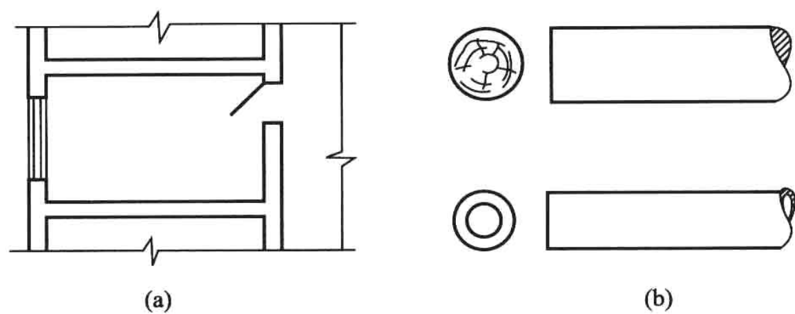
图 1 - 13 图形的折断 (a) 直线折断；(b) 曲线折断
