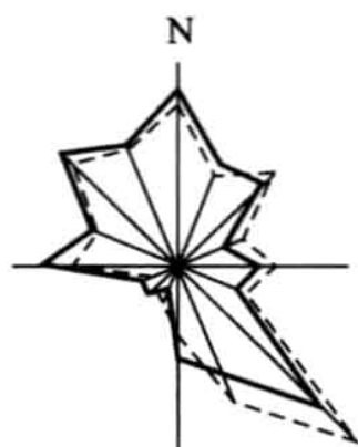
图 1-17 风玫瑰图
