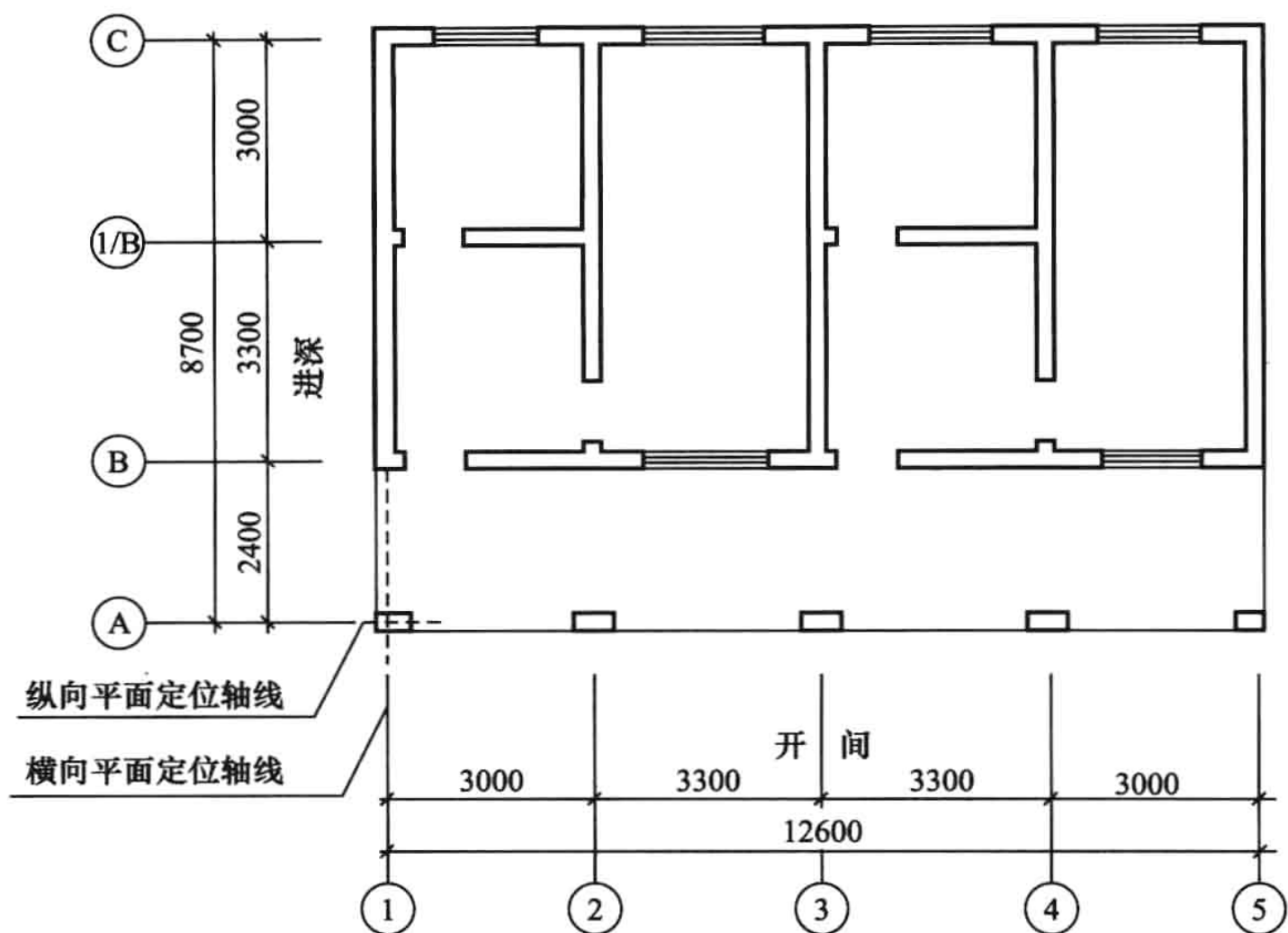
图 1 - 2 定位轴线编号方法
