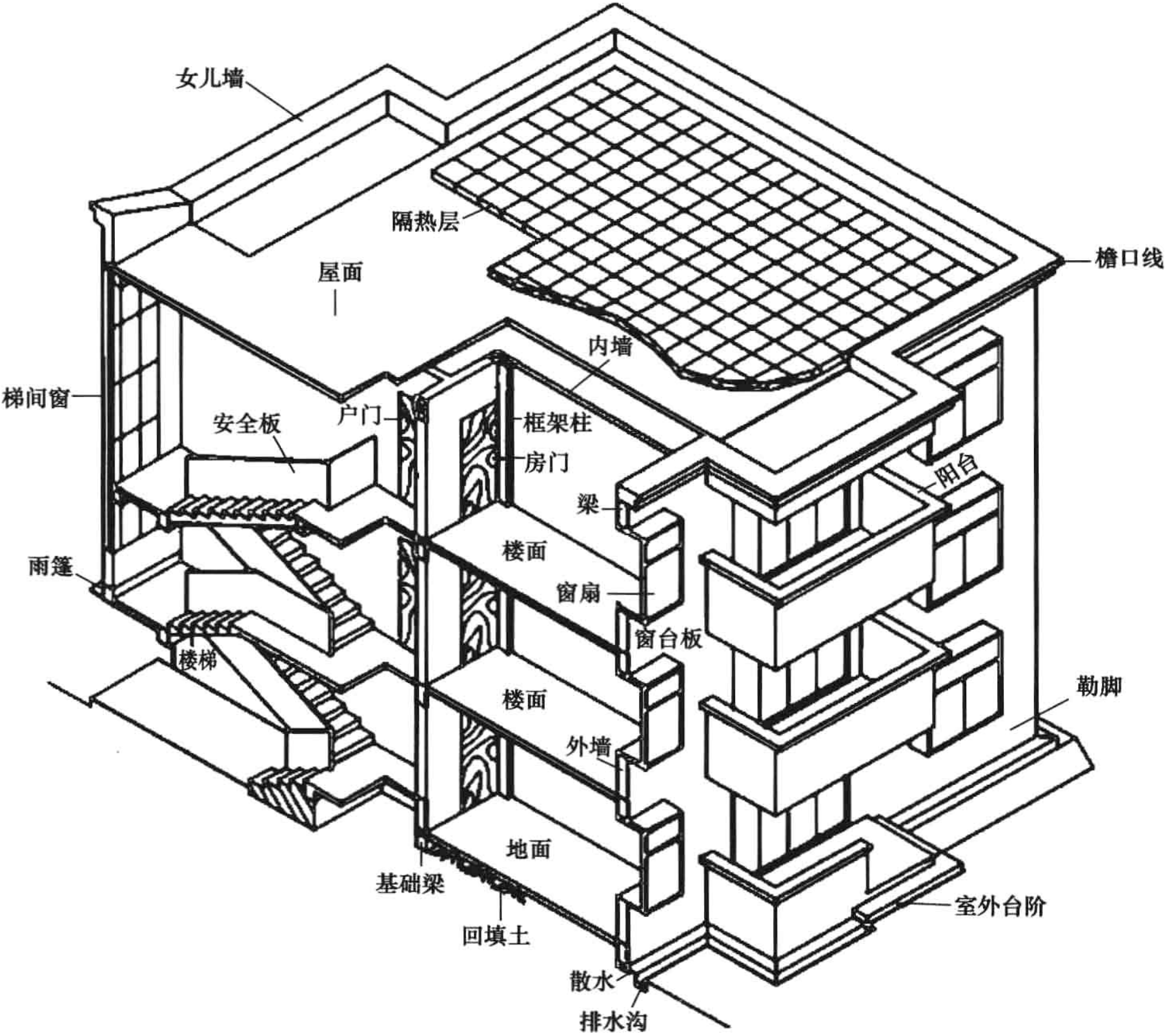
图 1-1 房屋的基本构成
