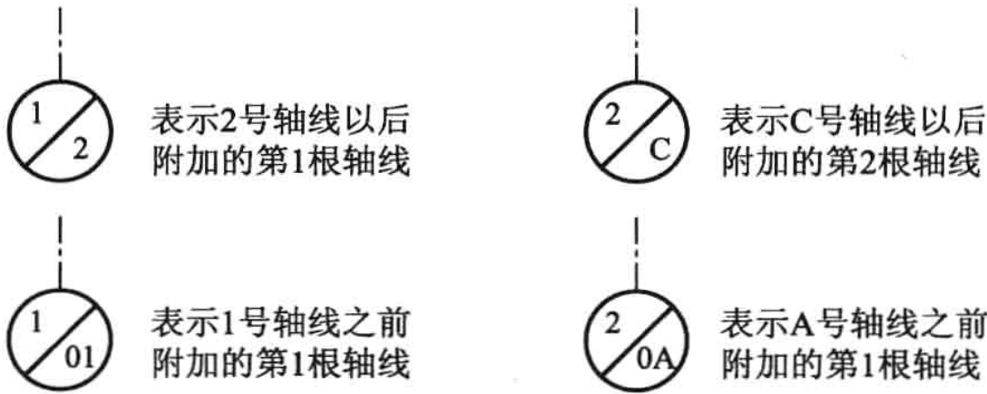
图 1 - 3 附加定位轴线的编号
