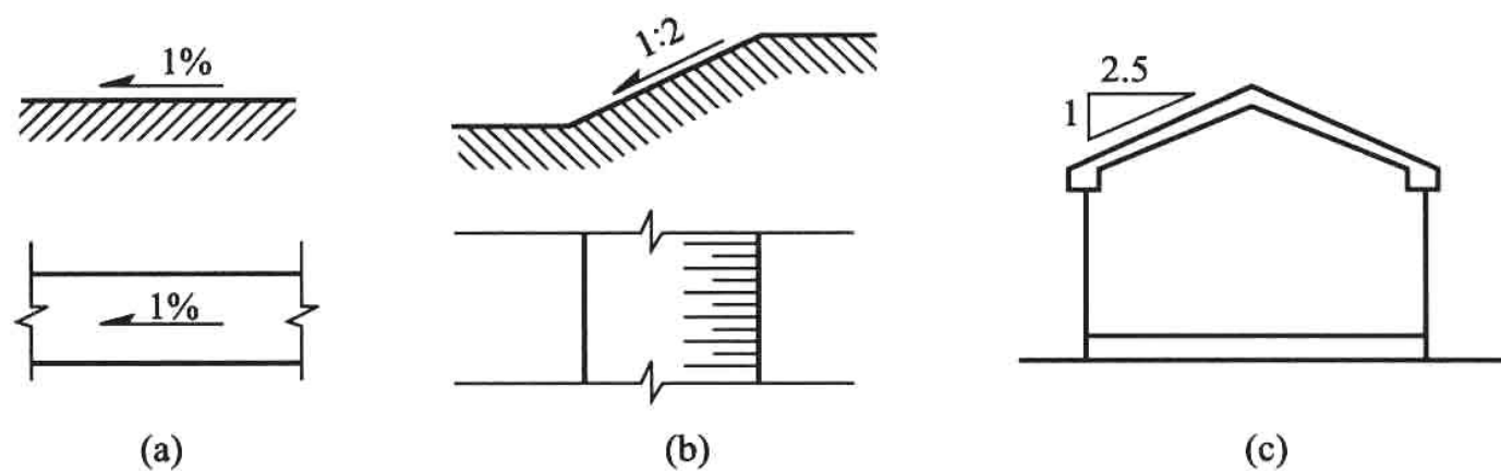
图 1 - 14 坡度标注方法
