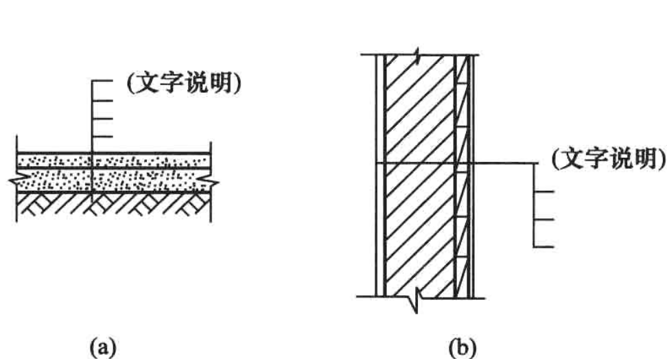
图 1-11 多层构造引出线
