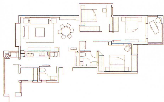
平面布置图
