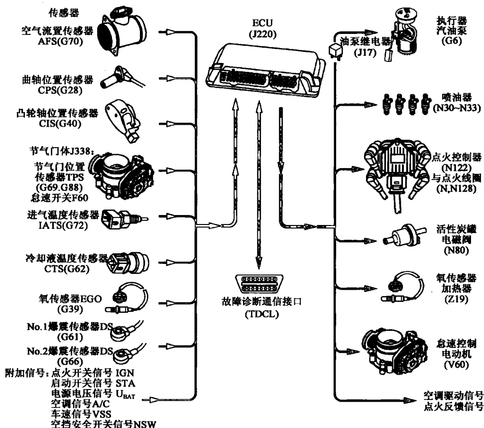
图 1-3 桑塔纳 2000GSi、3000 型轿车发动机电子控制系统的组成
