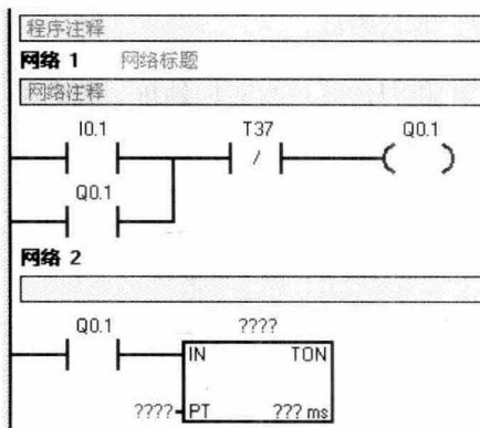
图 1-19 输入接通延时定时器
