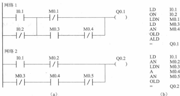
图 1-4 与块指令和或块指令的应用举例
