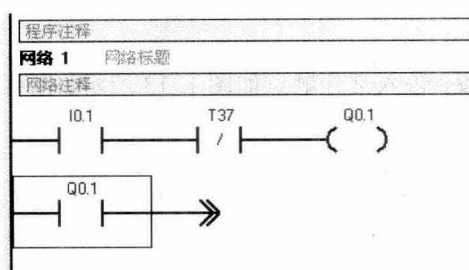
图 1-16 Q0.1 的编辑结果
