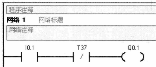
图 1-15 T37 和 Q0.1 编辑结果
