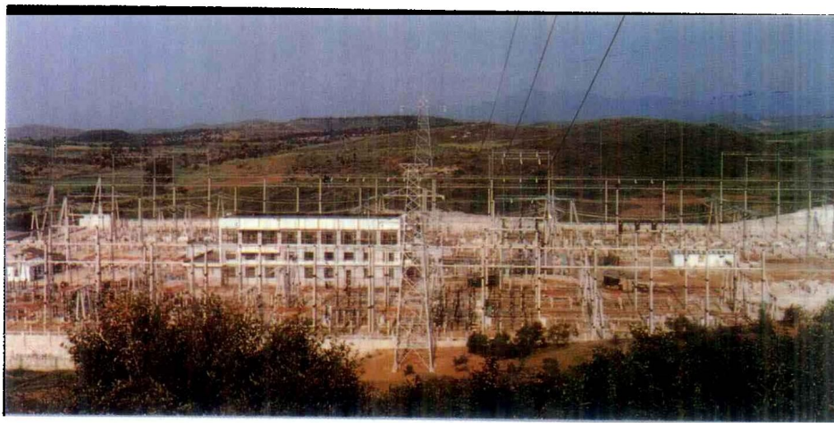
220 千伏凯里变电站外景。
