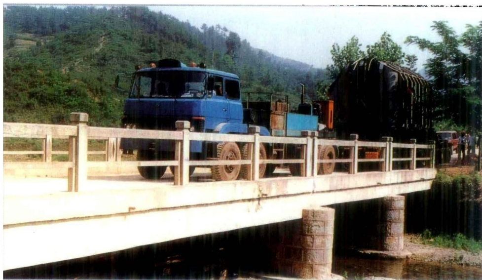
200 吨大型平板车运输变压器。
