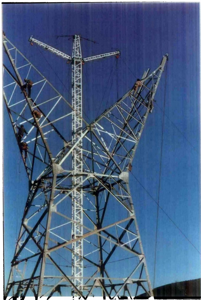
摇臂抱杆吊装工艺在铁塔组立中的应用。
