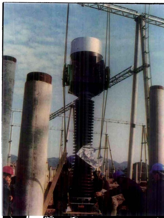
变电施工人员在贵阳 500 千伏变电站 吊装电流互感器。
