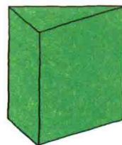
三棱柱
