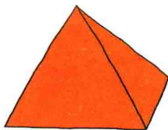
三棱锥
