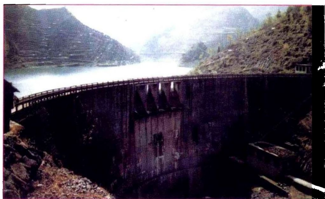
▲ 沿河官舟水库砌石双曲拱坝。坝高 64 米，总库容 2035 万立方米。
