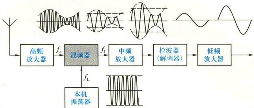
图 1.1.3 超外差式调幅接收机组成框图
