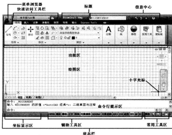
图 1-1 AutoCAD 初始界面
