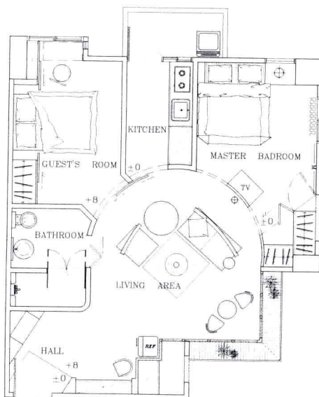
规划后平面配置图。
