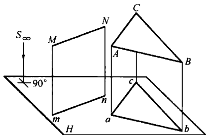
图 1-6 显实性
