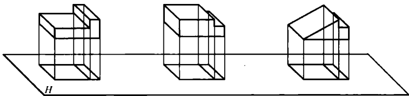
图 1-8 形体的单面投影
