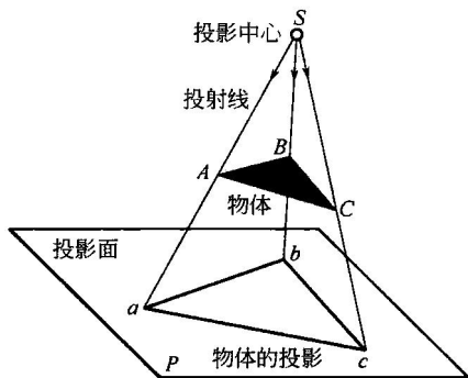
图 1-2 中心投影法
