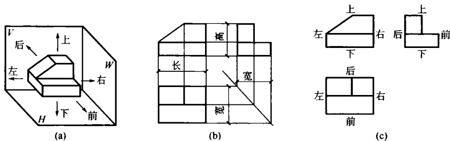
图 1-11 形体的方向
