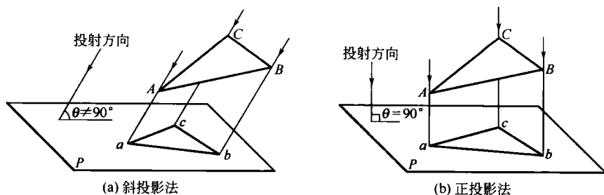
图 1-3 平行投影法
