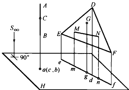
图 1-7 积聚性
