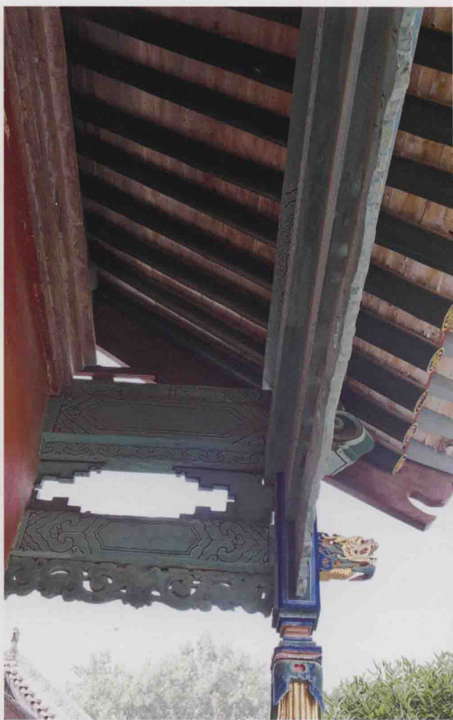
晋祠浮屠院挑梁梁架局部
