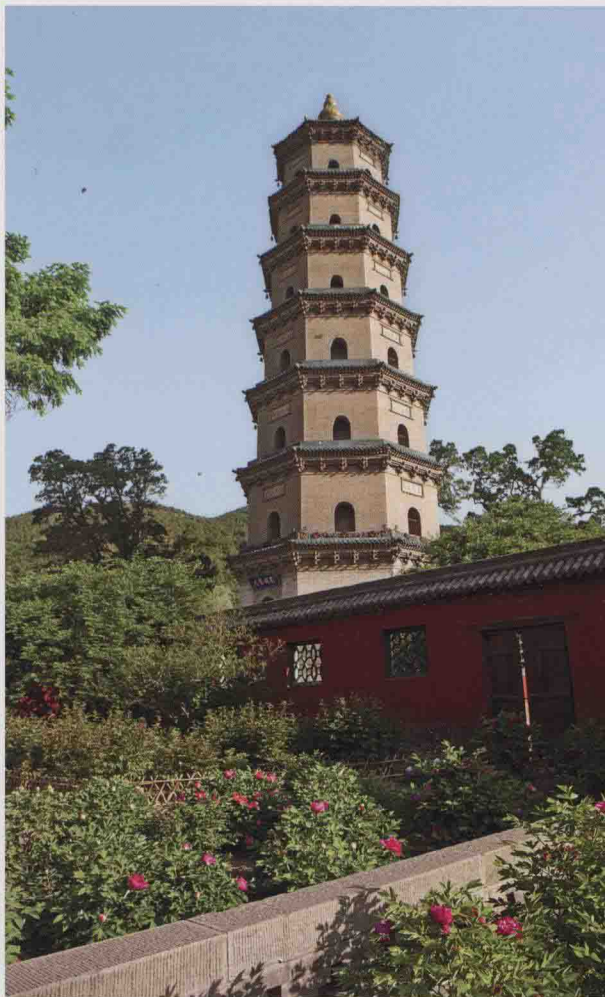
晋祠浮屠院舍利生生塔东南立面
