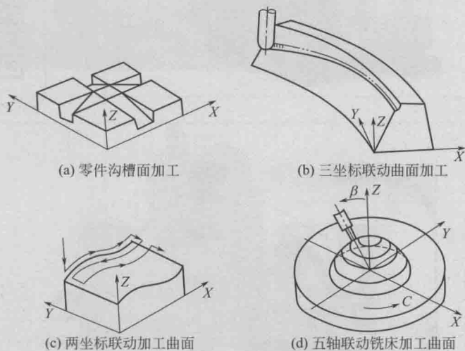
■ 图 1-3 空间平面和曲面的数控加工
