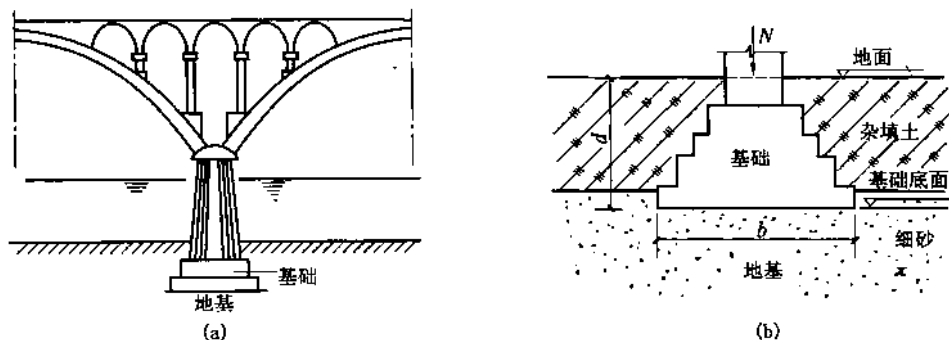
图 0.1 地基与基础
