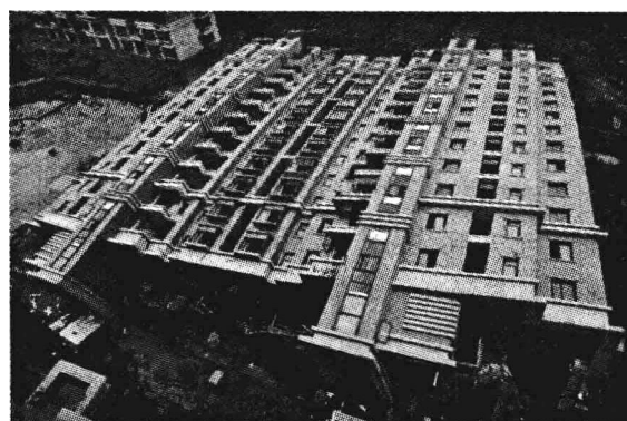
图 0.3 上海莲花景苑整体倒塌
