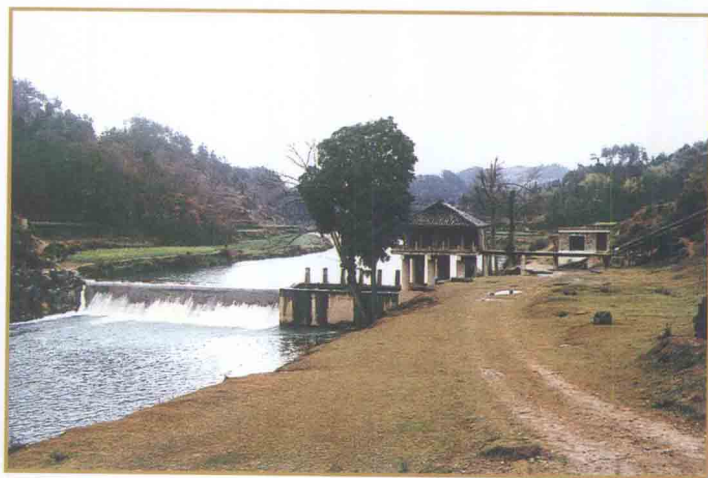
湄潭县核桃坝水轮泵站
