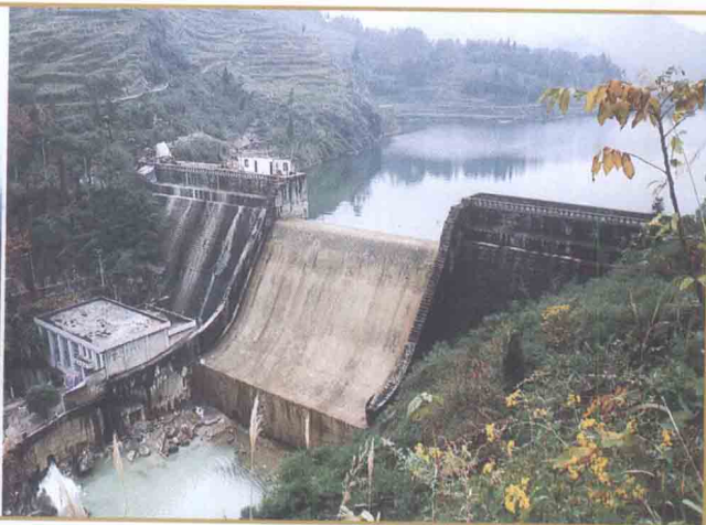
湄潭县湄江水库
