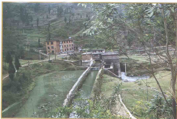
遵义县兰光水轮泵站
