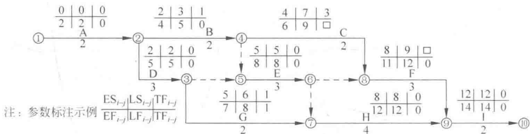
图 1-2 室内装饰装修工程进度计划网络图(单位:周)
